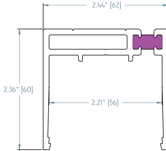
950WT HEAD / JAMB
