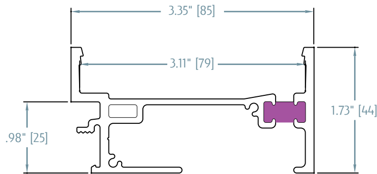
981WT SILL
