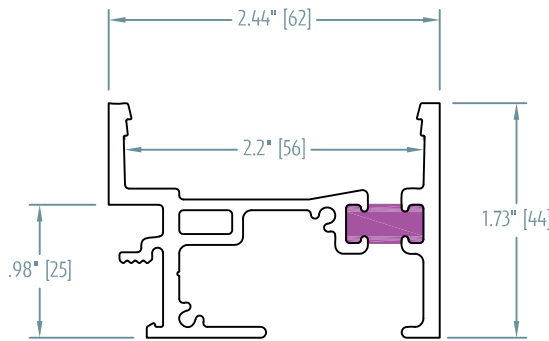
961WT SILL
